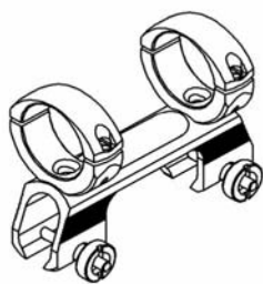
1. Винт крепежный 2. Охват 3. Винт стяжной 4. Гайка 5. Основание
