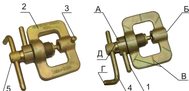
1 – прижим; 2 – корпус; 3 – винт стопорный; 4 – ключ-вороток; 5 – винт регулировочный; А, Д – риски; Б – отверстие; В – метки; Г – паз
