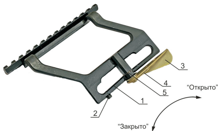
1 – основание; 2 - стопор; 3 – флажок; 4 - фиксатор; 5 – винт стяжной
